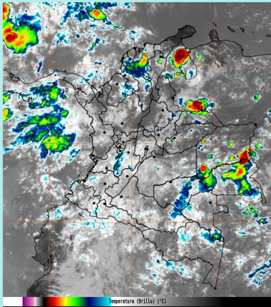
Imagen GOES 19 East Canal Infrarrojo, 7 de septiembre de 2025 - Hora 12:00 HLC. Fuente: IDEAM
